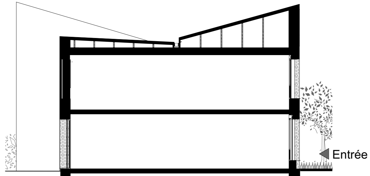
COUPE
