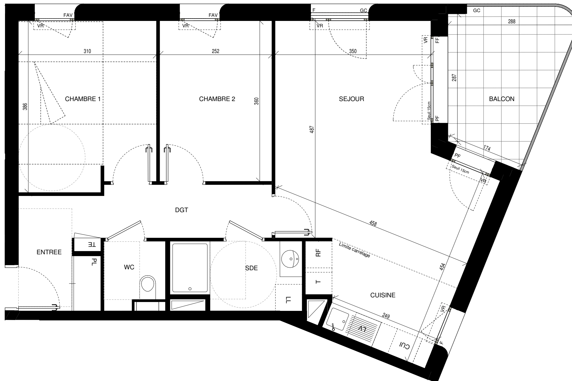
PLAN PROVISOIRE
