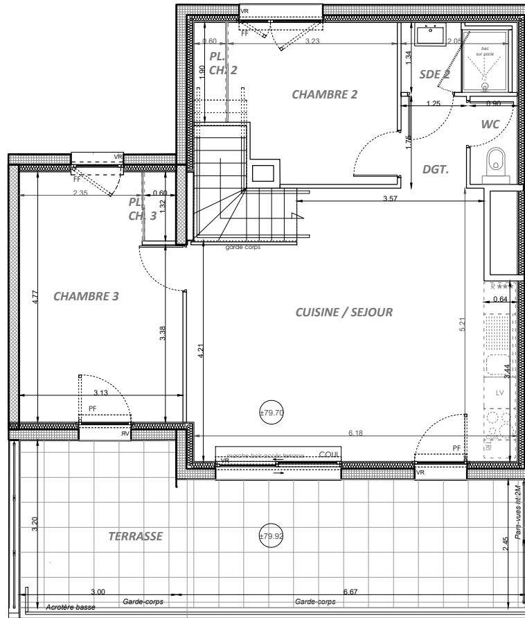
NIVEAU BAS DUPLEX (R+1)
