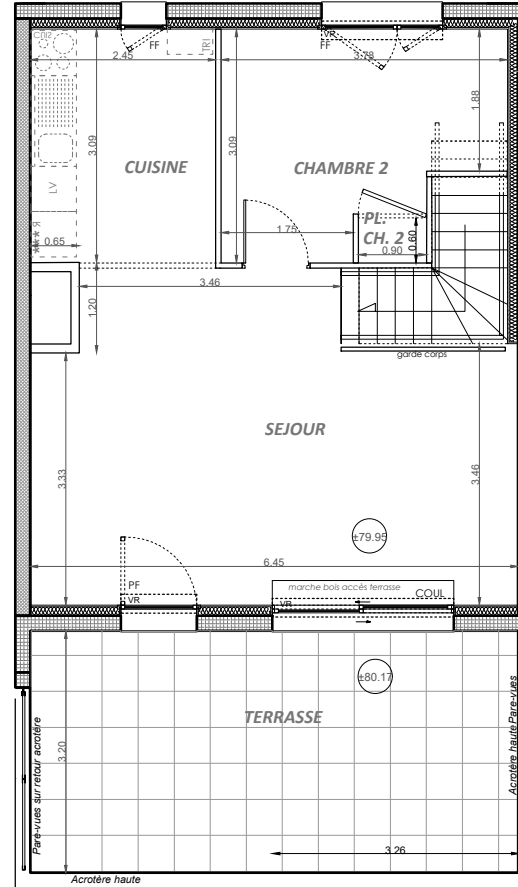
NIVEAU HAUT DUPLIX (R+2)
